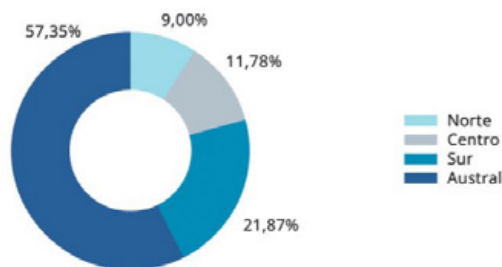
Gráfico 3.3.3 Total de glaciares a nivel nacional distribuidos por macrozona
